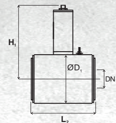
THREAD (EN 10226-1)
